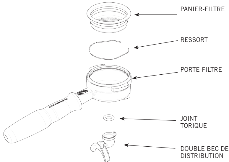
Figure 8 - Porte-filtre
