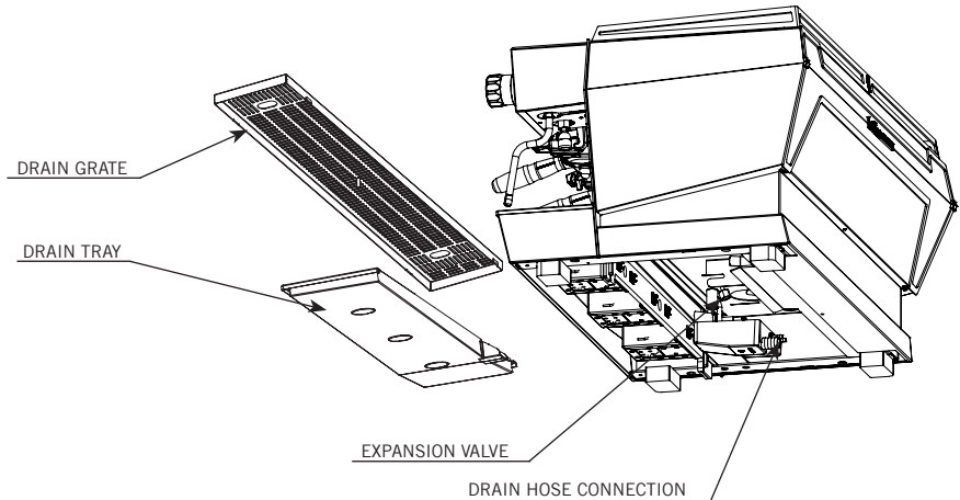
Fig. 3 - Installation Nomenclature
