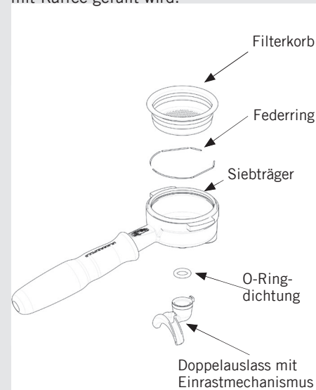
Abbildung 4 – Siebträger
