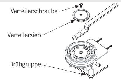
Abbildung 7 - Brühgruppensystem
